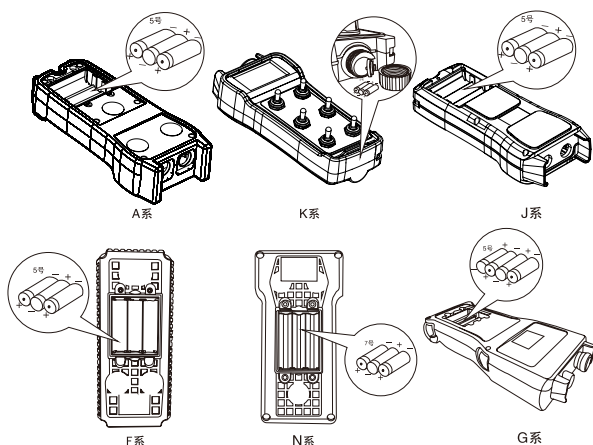
图3 (普通电池安装图)
