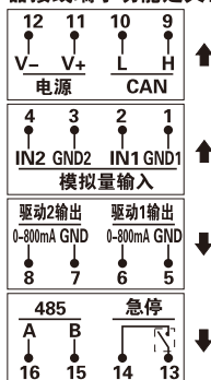
60系列—6080接收器接线端子功能定义:
